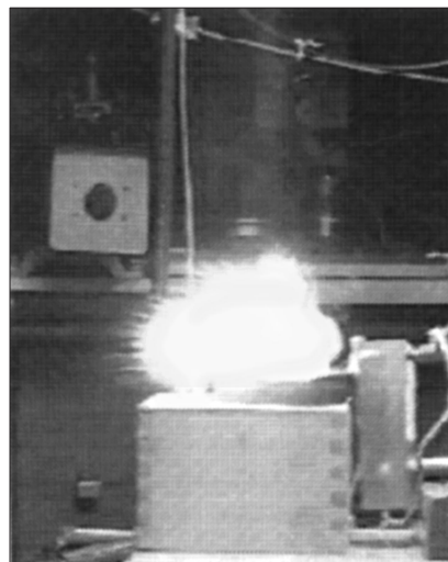
Рис. 4. Горение легкой фракции паров воска в результате взаимодействия с плазменной струей. Плазмотрон находится справа от ДСО.
